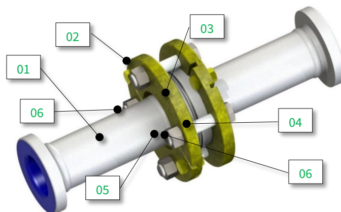
Bild 1: Stahl-Email-Flanschverbindung in ISO-Ansicht (Bildquelle: Düker)
